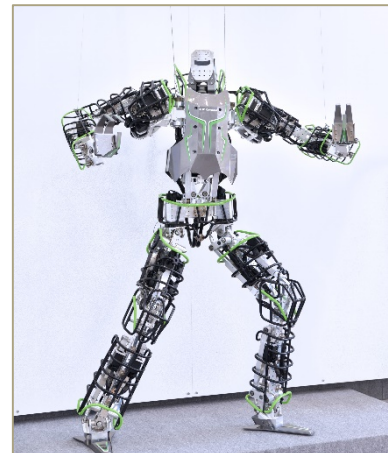
Humanoid robot Kaleido
